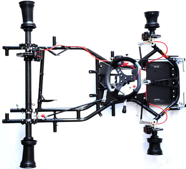
PHOTO VUE DE DESSUS DU CHÂSSIS COMPLET IDENTIQUE À L'UN DES MODÈLES PRÉSENTÉS À L'HOMOLOGATION SANS PARE-CHOC, CARROSSERIE, SIEGE, NI PNEUMATIQUES
